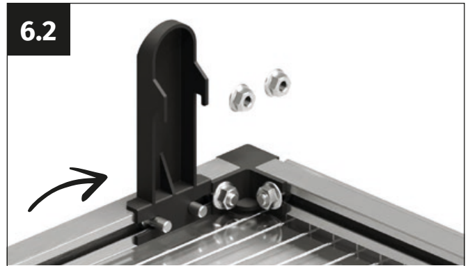
6.2 Positionieren Sie die Verschiebesicherung in den hinteren Ecken des Fensters an den seitlichen Fensterprofilen.
