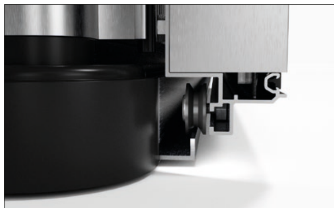
Detalje af den ophængte dør på den nederste dørskinne.
