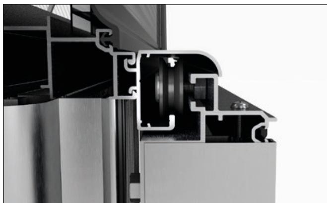
Detalje af den ophængte dør på den øverste dørskinne.
