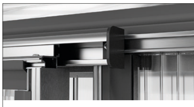
Fastgør dørskinnebeskyttelsen til dørskinnen. Skru dørskinnen fast med boreskruen, så dørskinnebeskytteren holdes fast i dørskinnens V-rille.
