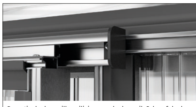
Bevestig de deurrailbeveiliging aan de deurrail. Schroef de deur-geleider vast met de boorschroef zodat de deurrailbeveiliging stevig in de rail wordt gehouden. Steek de boorschroef in de V-groef van de deurrail.
