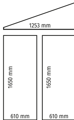
Zijwand - links
