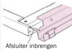
Afsluiter inbrengen
