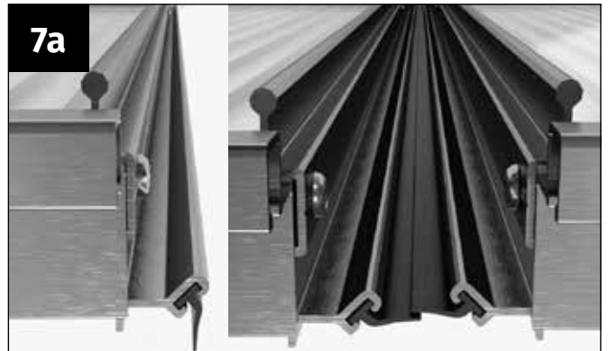
Detail Türdichtung seitlich
