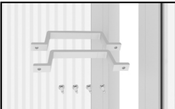
Tag dørhåndtag og de selvborende 4,8x13 mm skruer.
