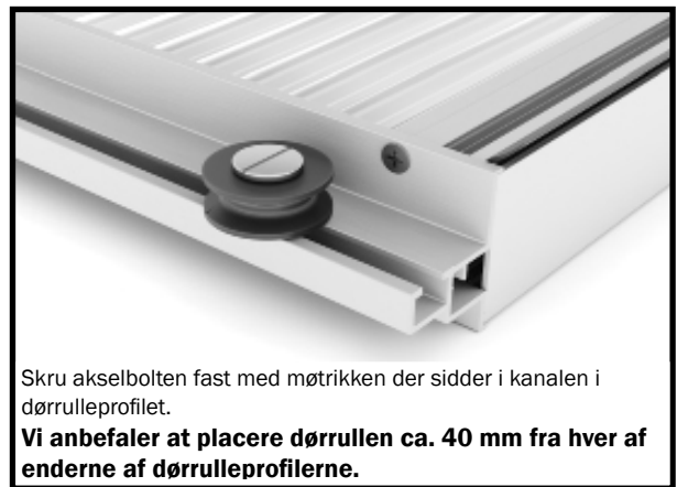
Indsæt M6 møtrikken i kanalen i dørrulleprofilen.
