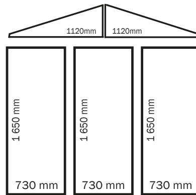
pignon avant
