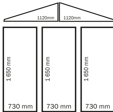
pignon arrière
