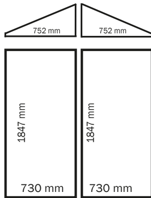
paroi arrière
