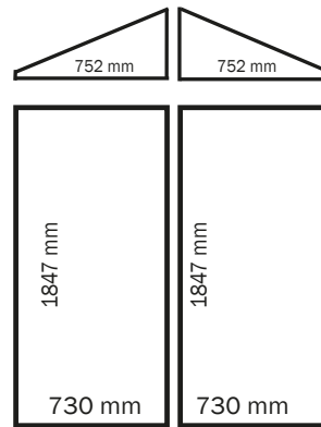
paroi avant
