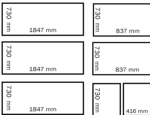
paroi arrière
